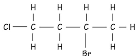
3-bromo-1-chlorobutane
